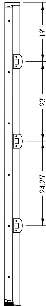
STRIKE JAMB
